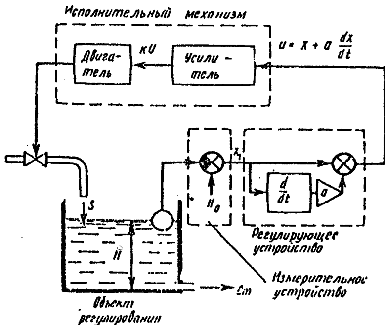
Рисунок. Схема системы автоматического регулювання рівня води в резервуарі
