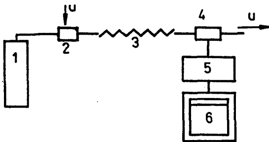
Рис. 1. Схема дослідницької установки з хроматографічною системою 1 – балон з несучим газом, 2 – дозатор, 3 – хроматографічна колона, 4 – детектор, 5 – електрометр, 6 – реєстратор, u – витрата газу-носія
