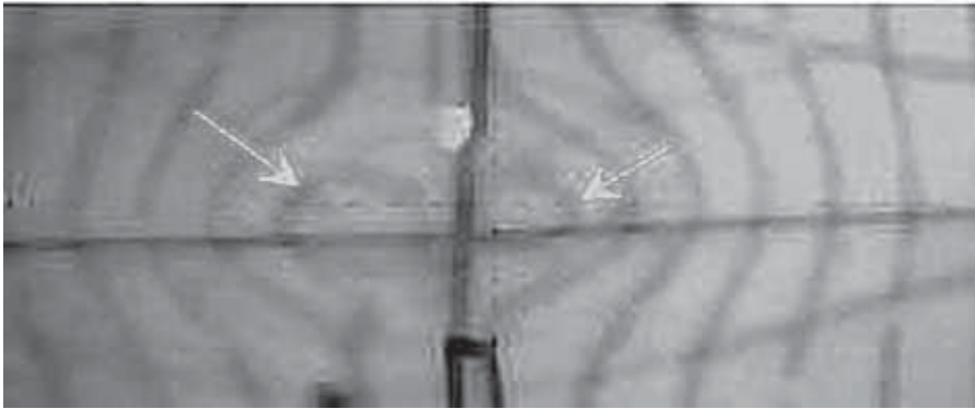
Рис. 2. Образование кольцевых структур (показаны стрелками) в слое воды толщиной 0,4 мм на поверхности бумаги
