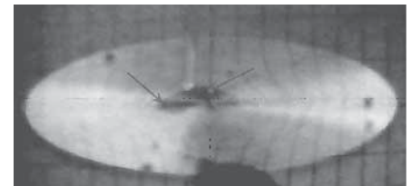
Рис. 3. Образование темных пятен.
