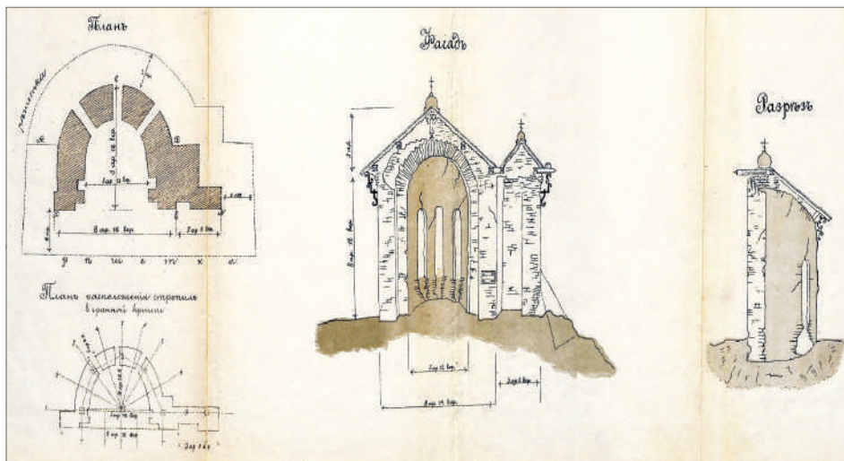
Кресленики Юр'євої божниці.
