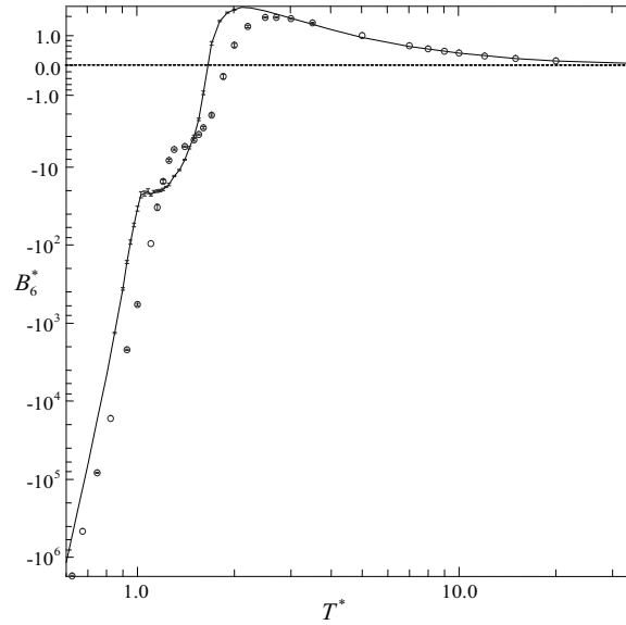
Рис. 2. Шестой вириальный коэффициент для mLJ потенциала. Вертикальные отрезки соответствуют погрешностям. Символы ( \circ ) показывают данные для LJ потенциала со своими погрешностями [26]
