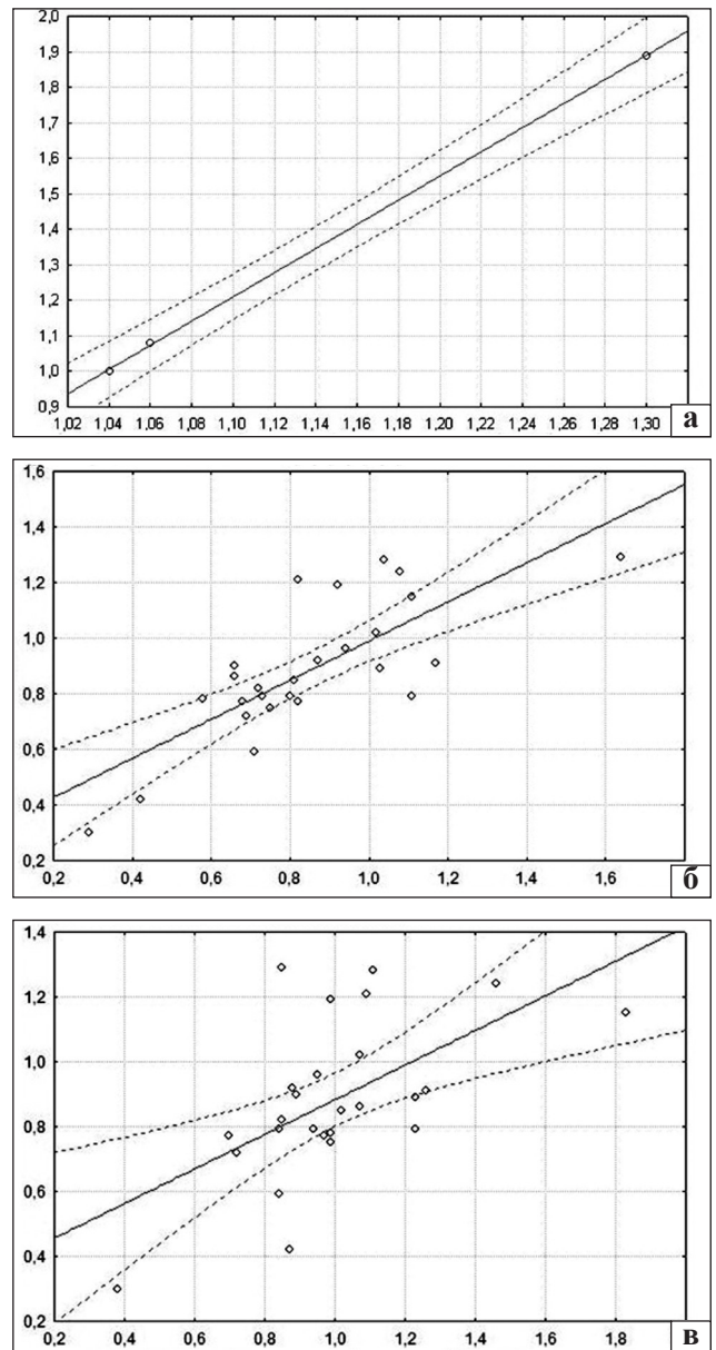
Рис. 3. Линии регрессии параметров ОЦМУ к ODI (а), VAS (б) и KST (в) в группах V_{\text{осн}} и V_{\text{контр}} через 3 мес. после операции — аппроксимированные кривые
