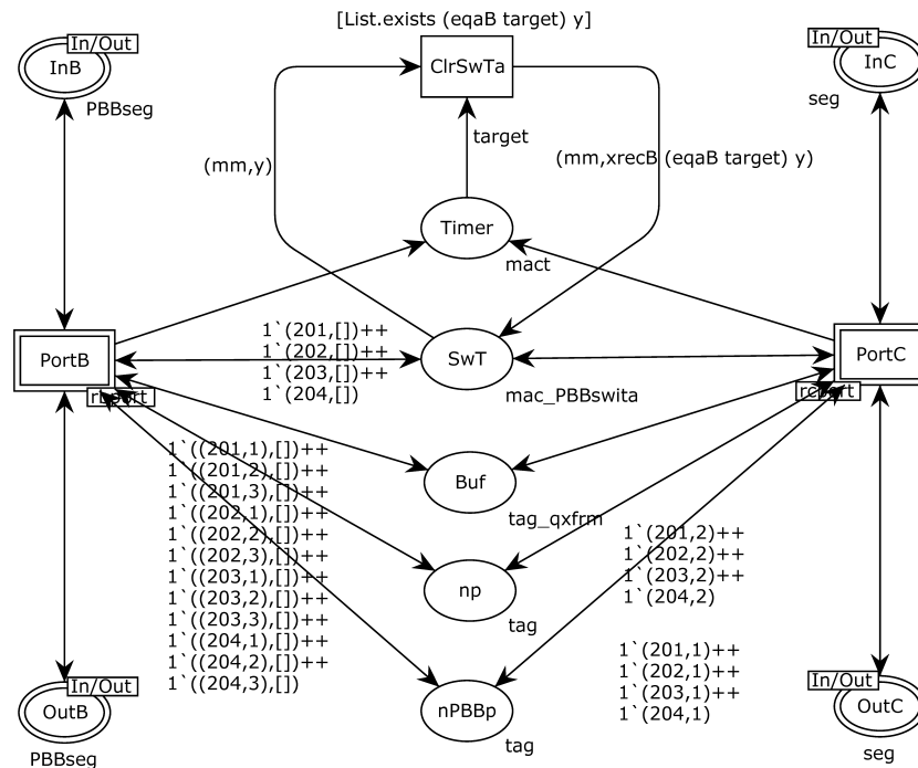
Рисунок 4 – Модель граничного PBB коммутатора
