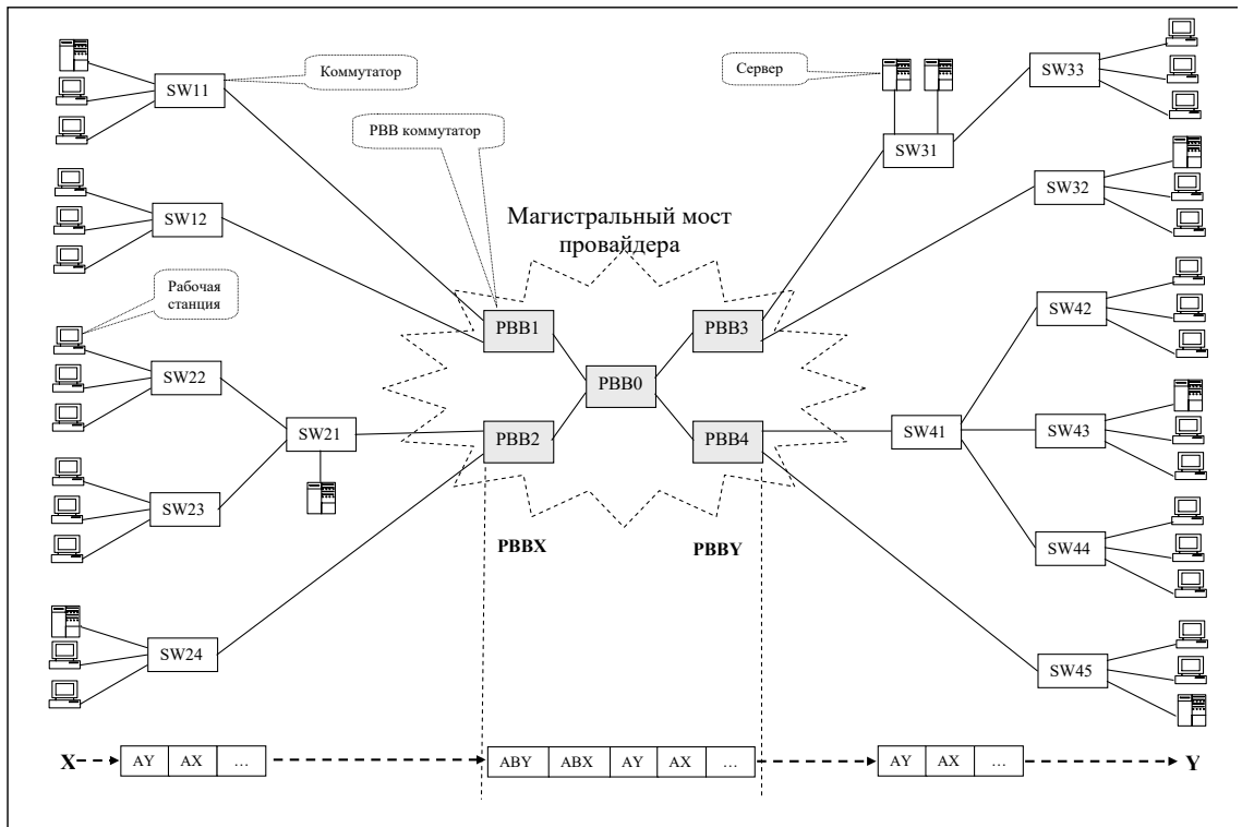
Рисунок 2 – Сеть с магистральным мостом провайдера PBB
