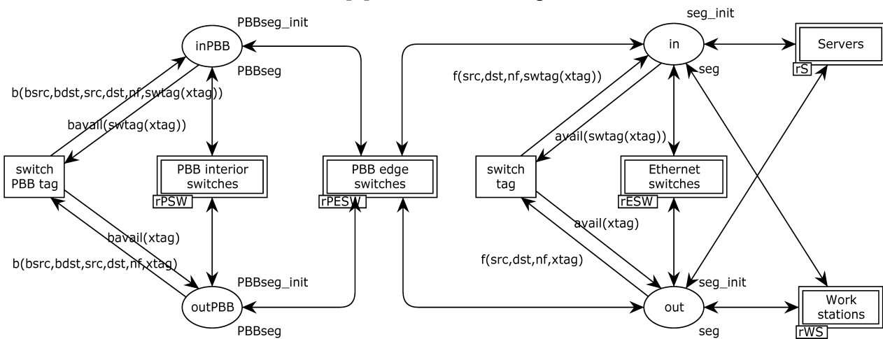
Рисунок 1 – Модель главной страницы РВВ сети
