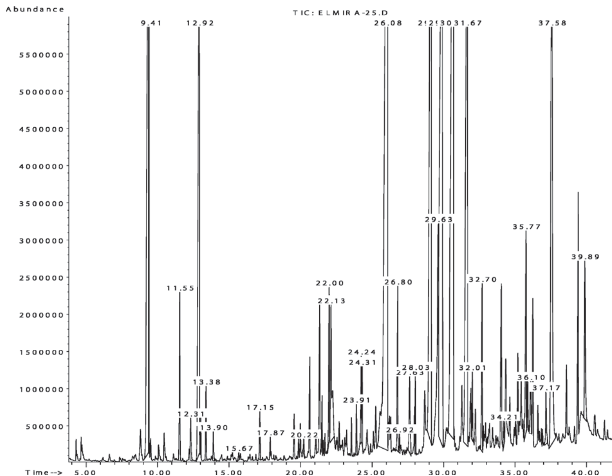
Рис. 1. Схема хроматограммы метиловых эфиров кислот травы ясенника распротертого
