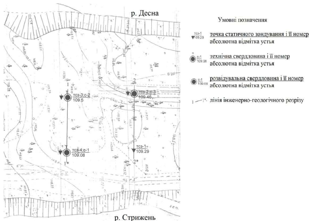
Рис. 1 – Схематичний план розташування виробок
