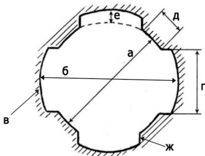
Рис. 13. Конструкція каналу ствола нарізної зброї.
