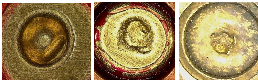
Рис. 2. Конструктивні відмінності відновленого ударника нейтралізованого пістолета Макарова (ліворуч) та штатного ударника аналогічної зброї (праворуч).
