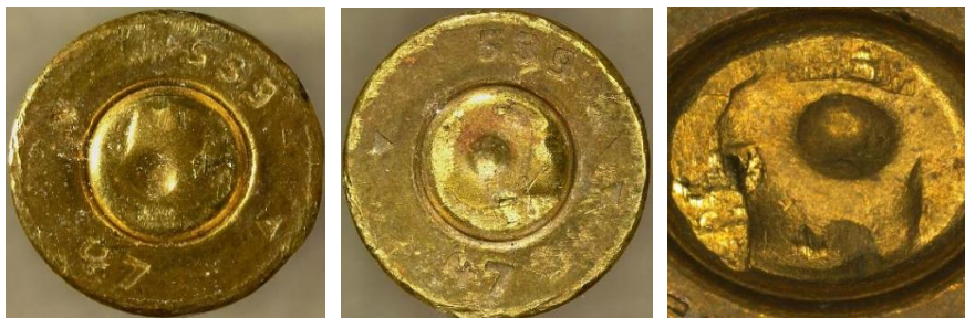
Рис. 6. Сліди зброї на гільзах, відстріляних з відновленої нейтралізованої зброї.
