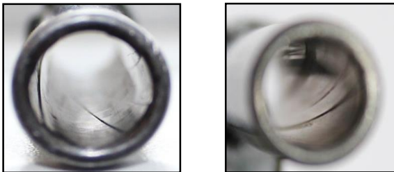
Рис. 16. Конструктивні відмінності каналу ствола саморобного виготовлення, встановленого на пістолет Макарова (ліворуч), та штатного ствола аналогічної зброї (праворуч).
