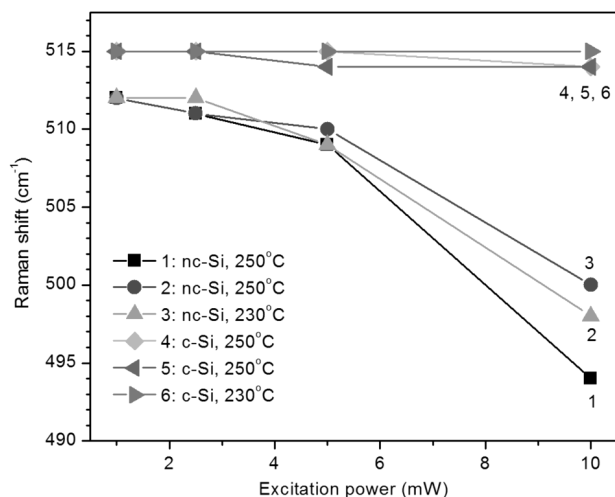
Рис. 11. Залежності частотного положення раманівських смуг нанокристалітів (1, 2, 3) та монокристалічної підкладки (4, 5, 6) при температурах 250\text{ }^\circ\text{C} (1, 2, 4, 5) та 230\text{ }^\circ\text{C} (3, 6) від потужності лазерного збудження
