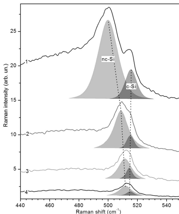
Рис. 9. Раманівські спектри структури c-Si/Sn(150 нм)/a-Si(50 нм), нагрітого до T = 250 \text{ }^\circ\text{C} , при зменшенні потужності P лазерного променя: 1 – P = 10 \text{ мВт} ; 2 – P = 5 \text{ мВт} ; 3 – P = 2,5 \text{ мВт} ; 4 – P = 1 \text{ мВт}
