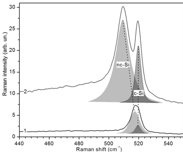
Рис. 10. Раманівські спектри структури c-Si/Sn(150 нм)/a-Si(50 нм), лазерно модифікованого при T = 250\text{ }^\circ\text{C} , P = 10\text{ мВт} , виміряні при T = 23\text{ }^\circ\text{C} і потужностях лазерного збудження P : 1 – P = 2,5\text{ мВт} ; 2 – P = 10\text{ мВт}
