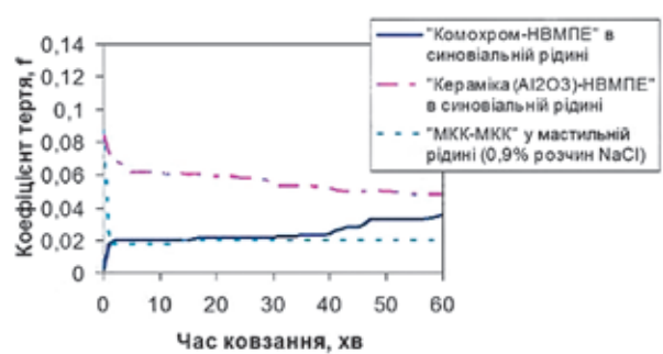
Рис. 6. Графік порівняння фрикційної поведінки коефіцієнтів тертя для різних пар матеріалів у синовіальній рідині та монокристалічній парі тертя у фізіологічному розчині NaCl
