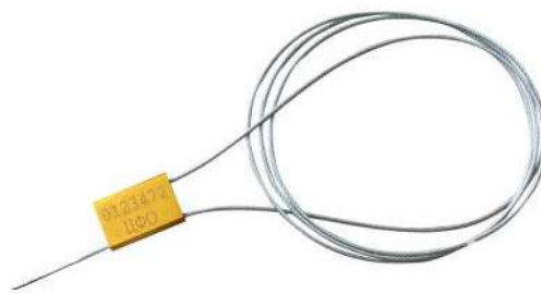
Силовий запірно-пломбувальний пристрій «СТРАЖ 2с»
