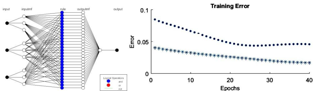
Рисунок 9 – Структурна схема мережі і графік результативності тренувань
