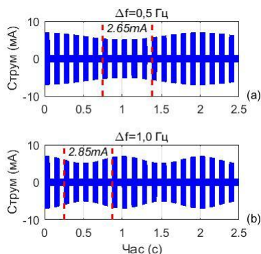
Рисунок 7 – Струм на вході КП ТРК в нормальному режимі при рівні гармонічної завади 0,7 мА
